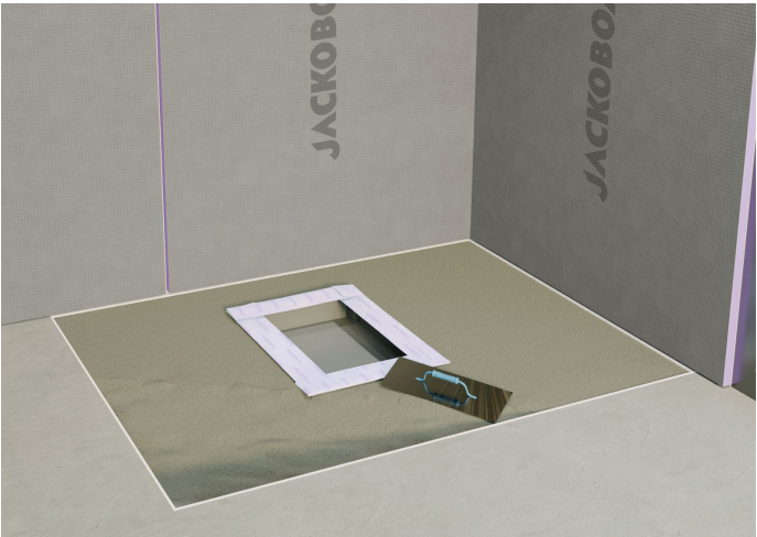
2) De vloeruitsparing vullen met egalisatiemortel
