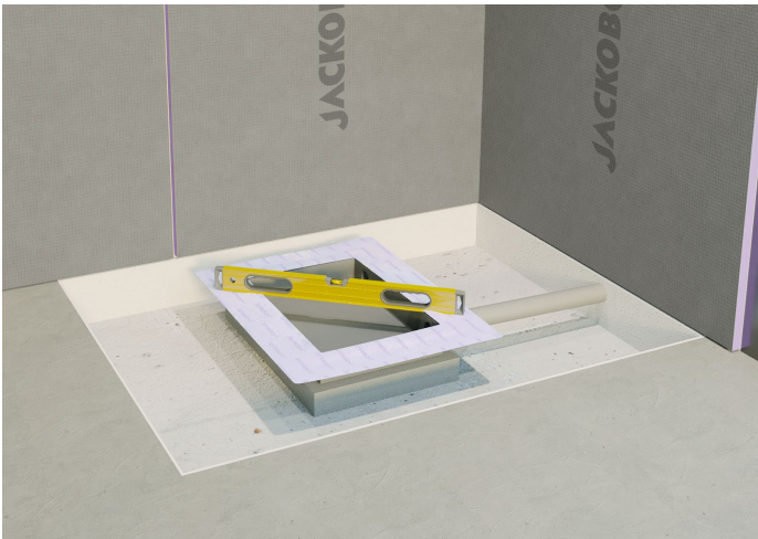
1) De installatiebox uitlijnen en aansluiten
